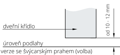
SVĚTLOST MEZI KŘÍDLEM A PODLAHOU
